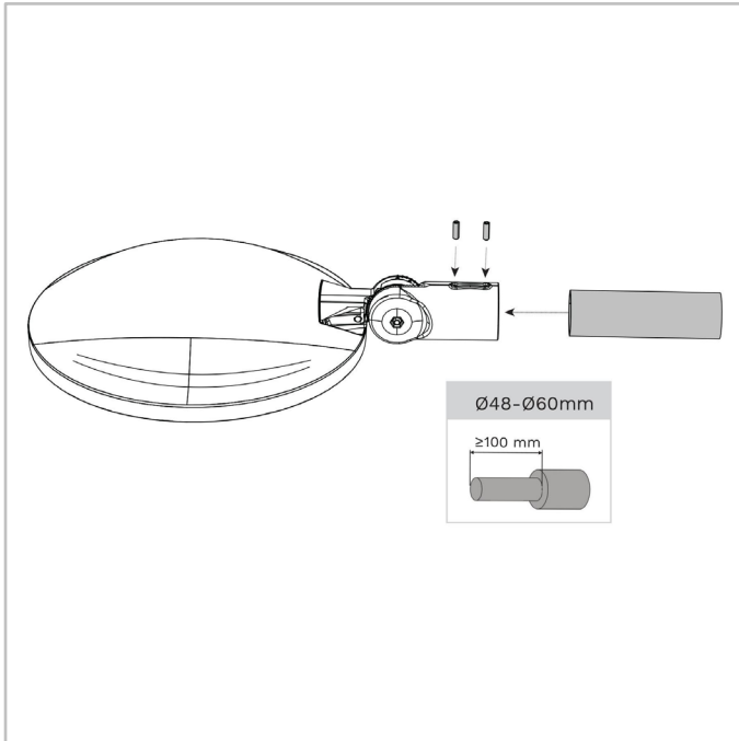
TOPIA | Mastansatzmontage für Zopf mit \varnothing 48-60 mm – 2 x M8-Schrauben
