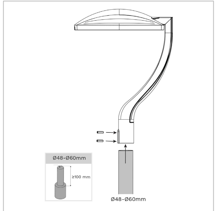
TOPIA | Mastaufsatzmontage auf Zopf mit \varnothing 48-60 mm
